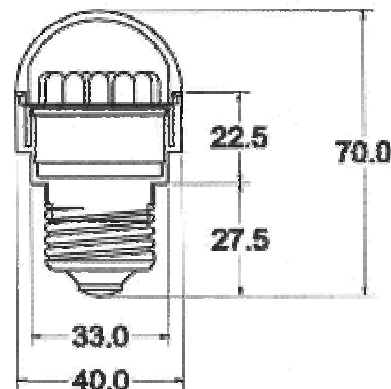
E27 Screw cap
